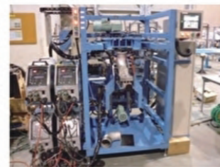
●多電極溶接装置
