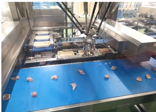
←唐揚げ用のお肉を自動でトレーに盛り付ける機械
