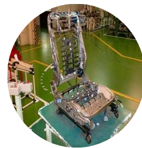
④～⑤ フレーム締付け工程
