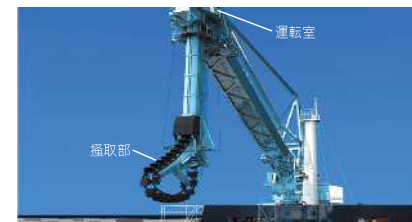
連続アンローダ全景
