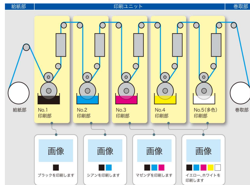
図2 重ね塗り工程
