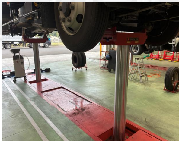
2柱リフト
